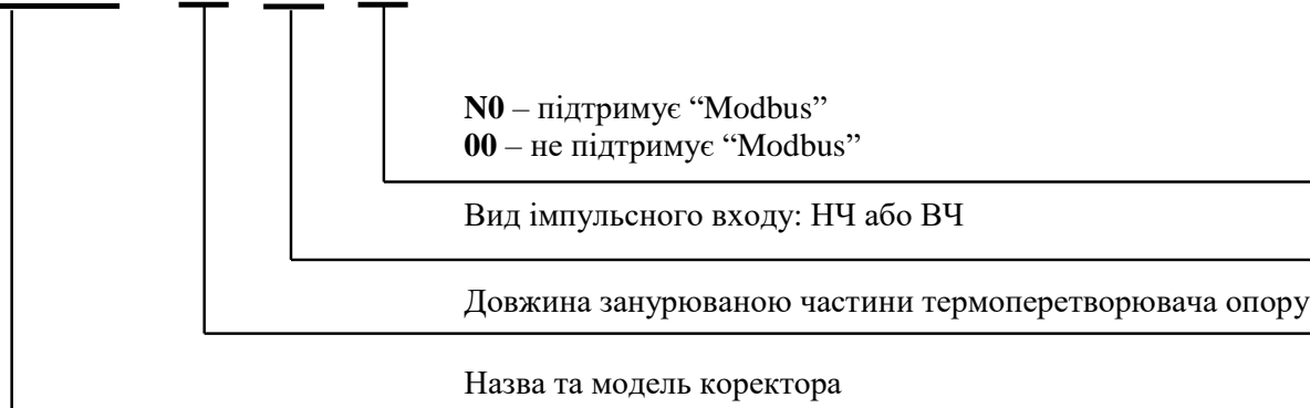
Рисунок 1 – Схема складання умовного позначення коректорів ВЕГА-2.01
